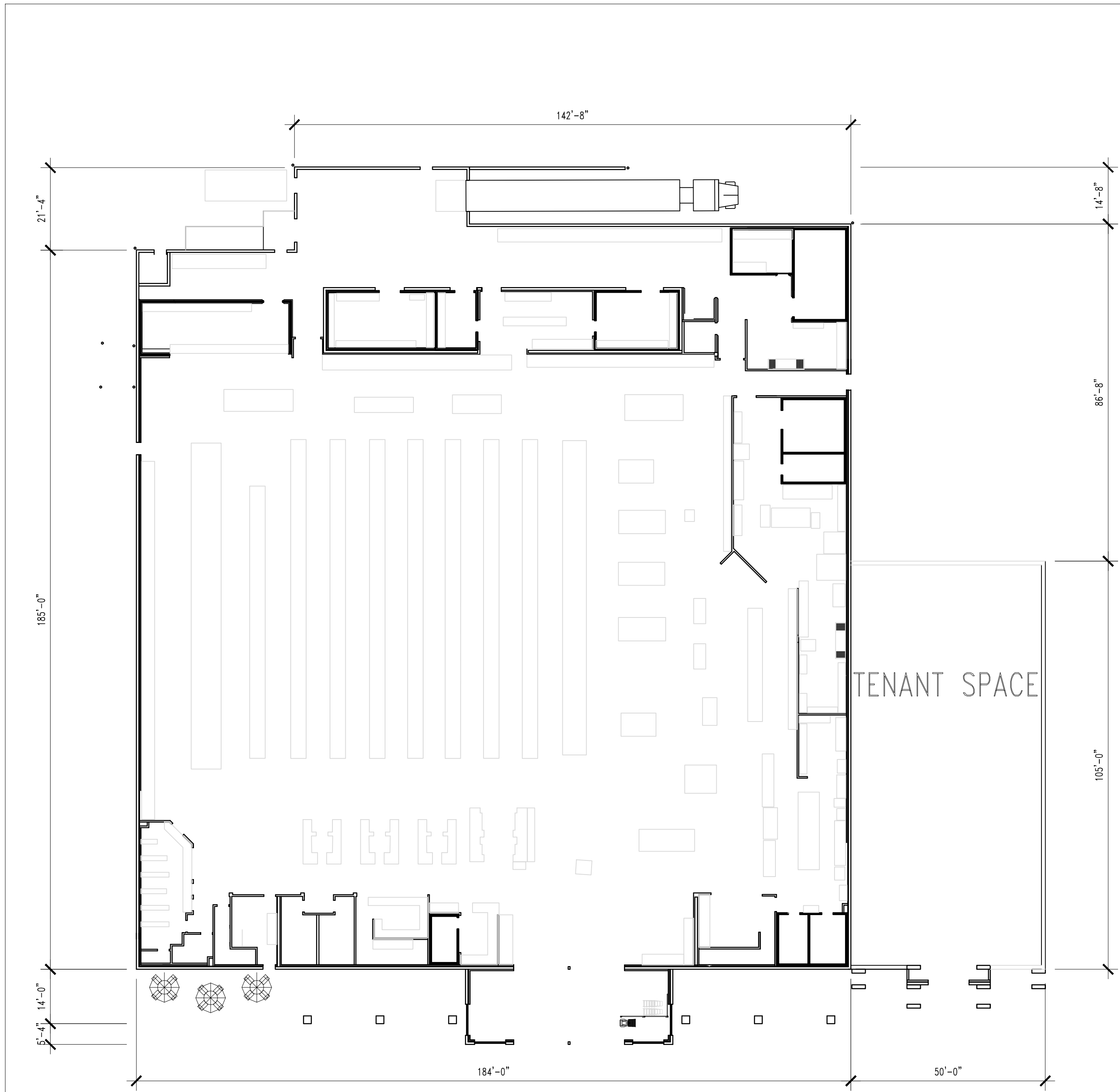
GROCERY & TENANT SPACE
